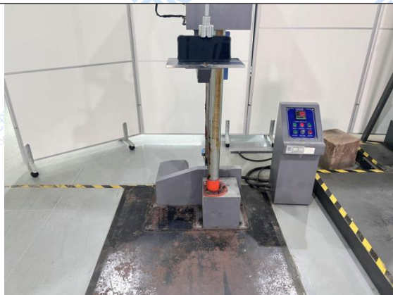
Fig.69 Test setup- Edge (3)
