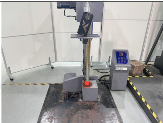
Fig.78 Test setup- Edge (12)
