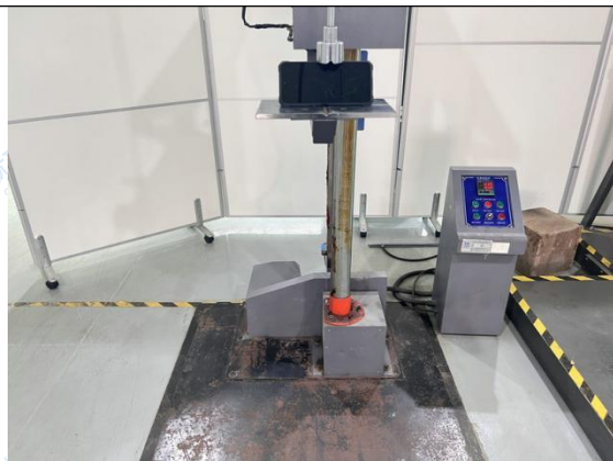
Fig.68 Test setup- Edge (2)
