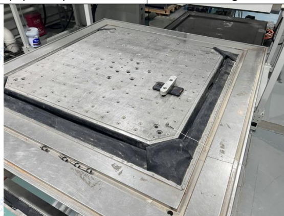
Fig.43 Test setup (Z axis)
